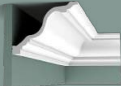
C334 | C334F 200 x 15 x 19,6 cm Purotouch® 19,6 15 ∇ = 24,1
