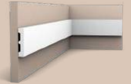
SX157 | SX157F SQUARE 200 x 6,6 x 1,3 cm Duropolymer ®
