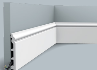
SX118 | SX118F | SX118-RAL9003 CONTOUR 200 x 13,8 x 1,8 cm Duropolymer®
