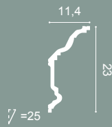
4 C332 200 x 23 x 11,4 cm Purotouch®
