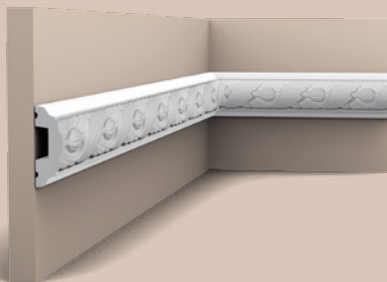
P1020 200 x 4,9 x 2,4 cm Purotouch®
