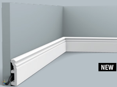
1 SX195 | SX195F HAMBURG 200 x 8 x 1,9 cm Duropolymer®
