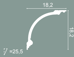
2 C338 200 x 18,2 x 18,2 cm Purotouch®
