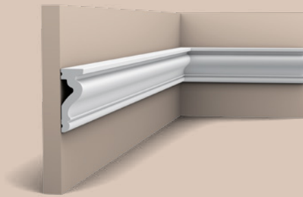
1 DX174-2300 | DX174F 230 x 6 x 2,2 cm (DX174-2300) Duropolymer® 200 x 6 x 2,2 cm (DX174F)
