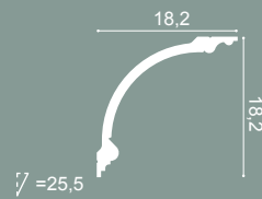
3 C338B BA'ROCK 200 x 18,2 x 18,2 cm Dessin: 2 x 57 cm Purotouch®
