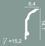
C339 | C339F 200 x 14,1 x 6,4 cm Purotouch®
