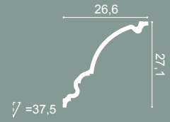
C336 200 x 27,1 x 26,6 cm Purotouch®
