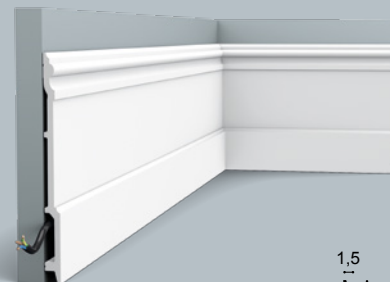
3 SX191 HIGH RISE 200 x 21 x 2,1 cm Duopolymer®
